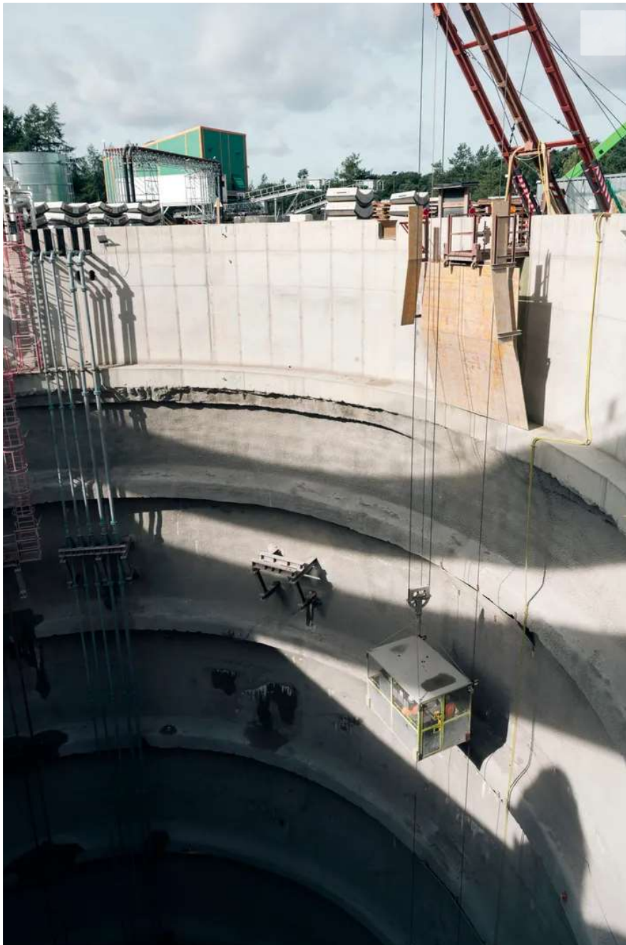
Einfahrt zum Grubenwasserkanal: Mega-Baustelle mitten im Wald Foto: Jan Richard Heinicke / DER SPIEGEL
